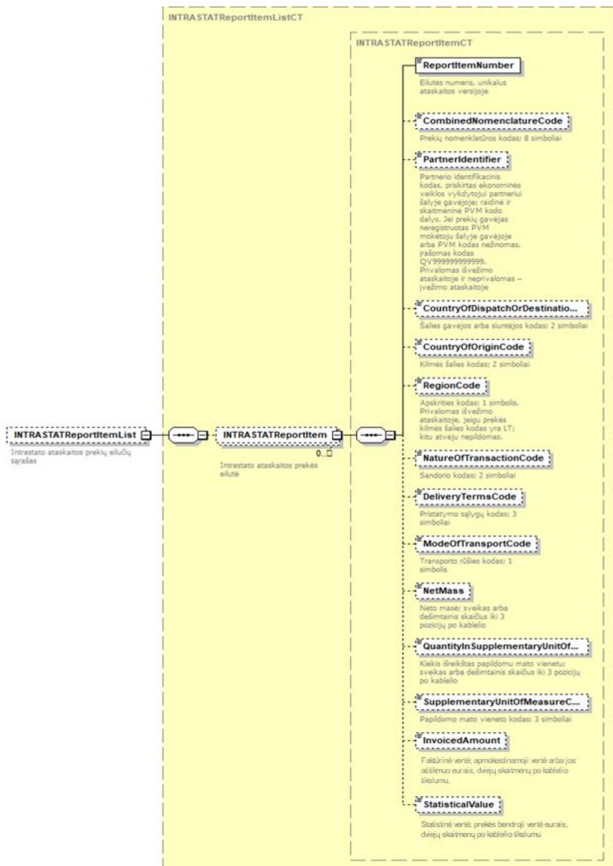
10 pav. Ataskaitos prekių sąrašo schema
