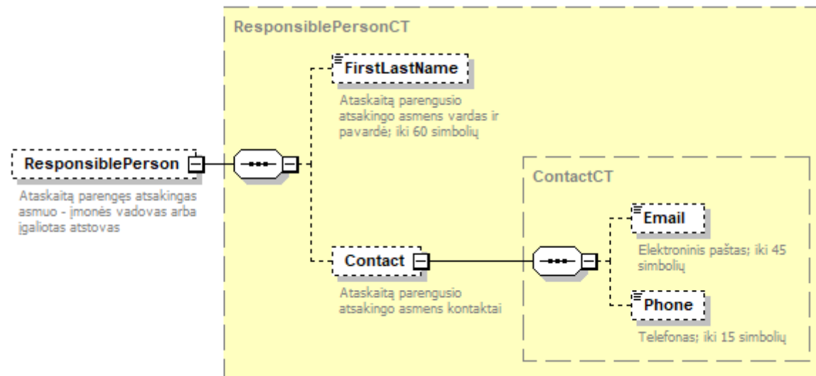
8 pav. Parengusio asmens schema
