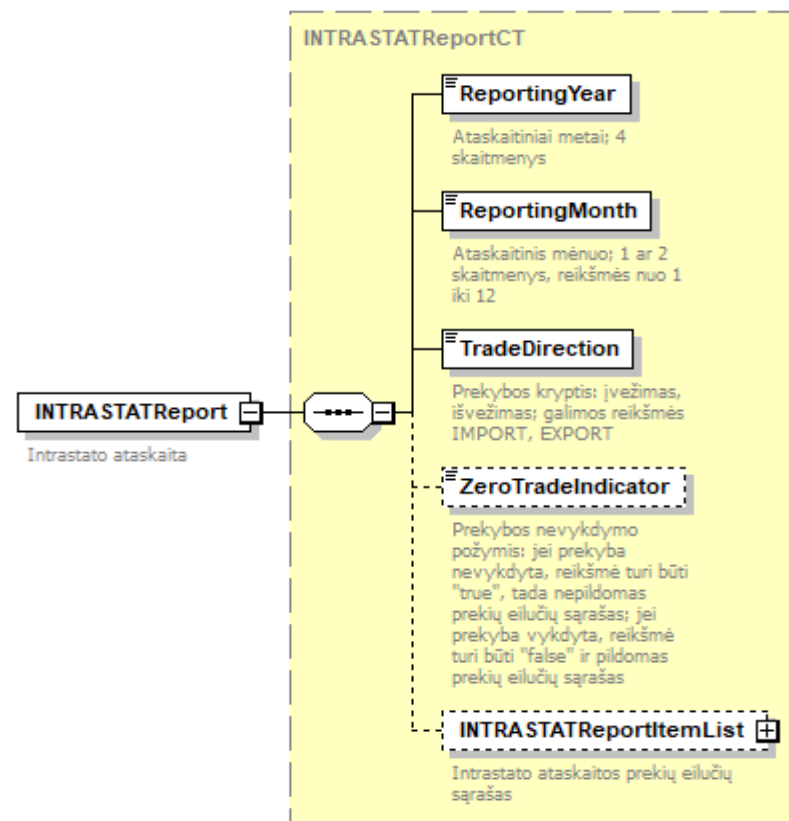
9 pav. Ataskaitos bendrosios dalies schema
