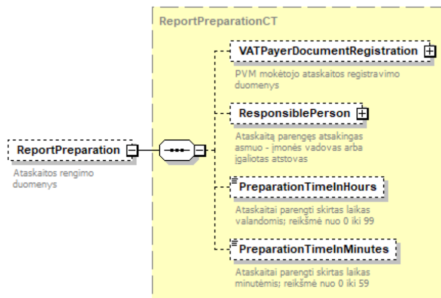
6 pav. Ataskaitos rengimo schema
